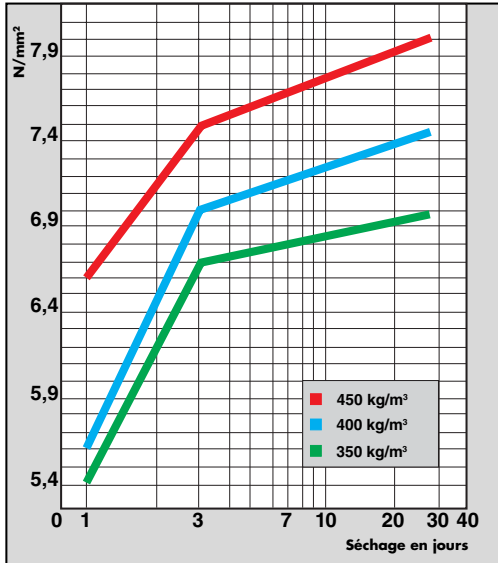
RESISTANCE A LA FLEXION DE MAPECEM A DIVERS DOSAGES
